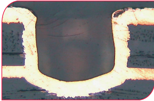
Blind Via mit zylindrischem Werkzeug
